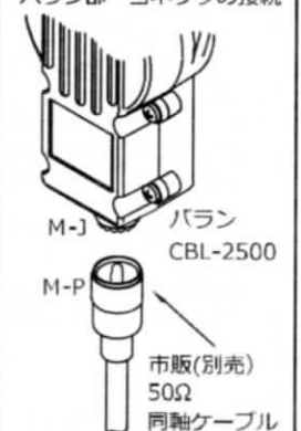
【図3】 バラコ部 コネクタの接続
