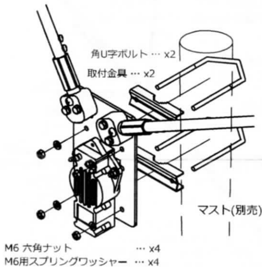
【図2】 金具2セットの取付
